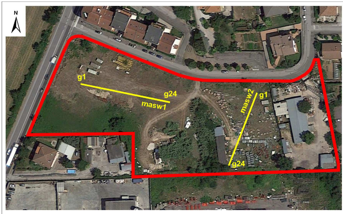
Ubicazione delle prove sismiche (base estratta dalle mappe di Google Maps)
