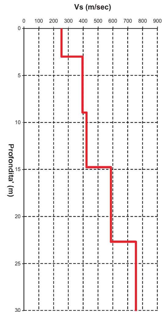
Profilo verticale onde S
